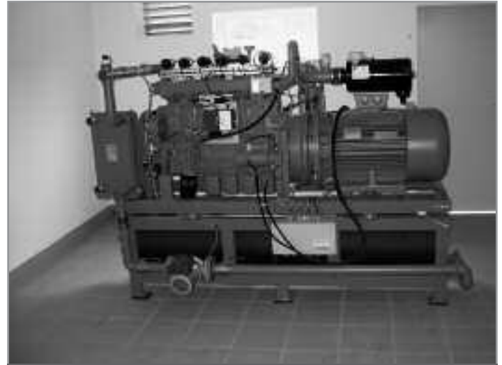
Das »Kraftwerk«: links der Motor und rechts der Generator
